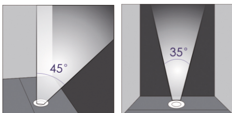
Soczewka/Lens angle 45/35°
